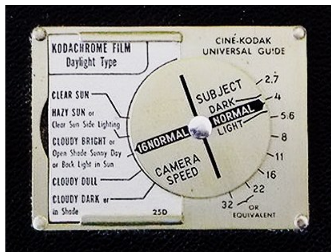
Figure 21. Ciné-Kodak Universal guide
